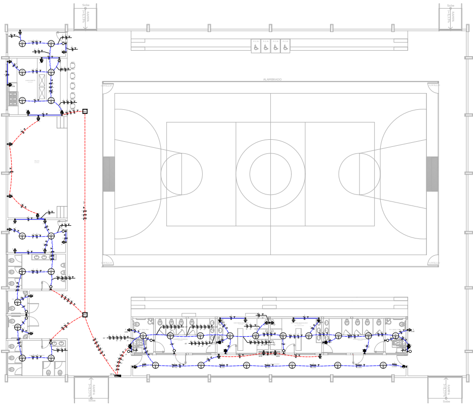
03 PLANTA BAIXA DE ILUMINAÇÃO E TOMADAS ESCALA 1:10
