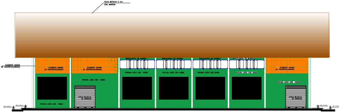
FACHADA ESCALA 1/75
