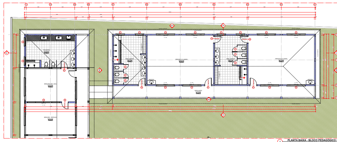
1 PLANTA BAIXA - BLOCO PEDAGÓGICO
