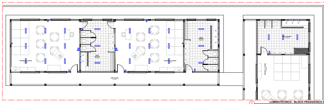
LUMINOTÉCNICO - BLOCO PEDAGÓGICO C
